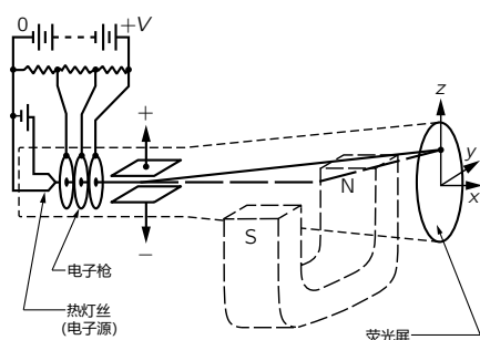
图 12.3: 电子束管
