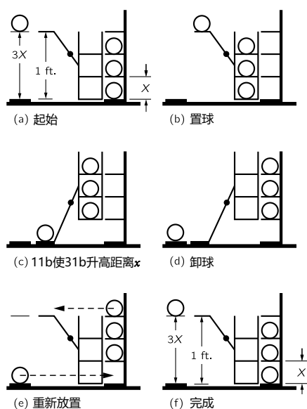
图 4.2: 一种可逆机
