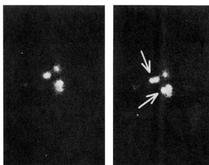
图 7.12: 新星的形成
