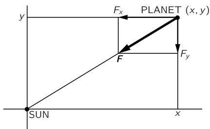
图 9.5: 作用在行星上的太阳引力
