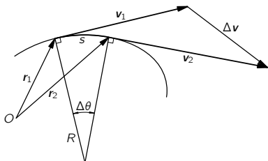
图 11.7: 曲线轨道示意图
