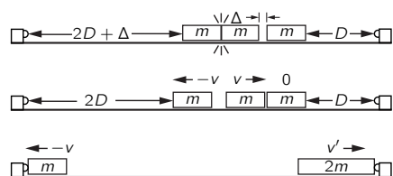
图 10.6: 验证以速度 v 运动的质量为 m 的物体与一个质量相同的静止物体碰撞后结合在一起以质量 2m 、速度 \frac{v}{2} 运动的实验
