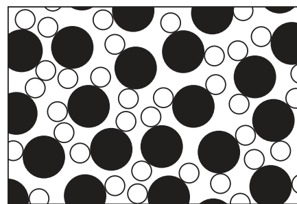
图 1.1: 放大 10 亿倍的水
